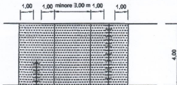
figura 5 scavi multipli
