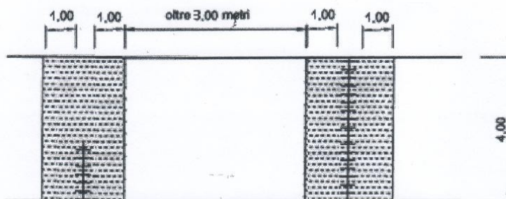
figura 6 scavi multipli
